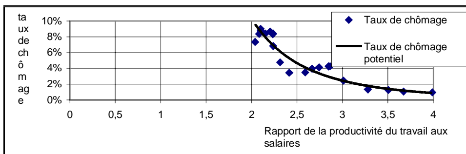
Figure 31. Relation entre le rapport de la productivité du travail aux salaires et le taux de chômage (1965–1990)
